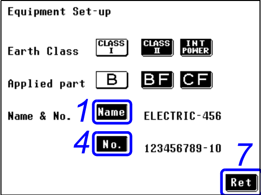
测试设备的设置画面
