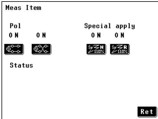
例：用于网络 B2 和患者泄漏电流（金属可接触部）测量的自动测量项目设置画面
