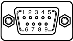
带有 M2.6 固定螺丝的 D-sub 9 针公头连接器
