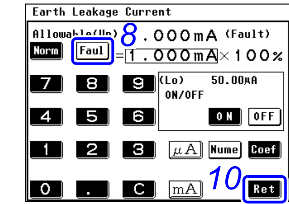
容许值设置画面 (故障状态，数值设置模式)
