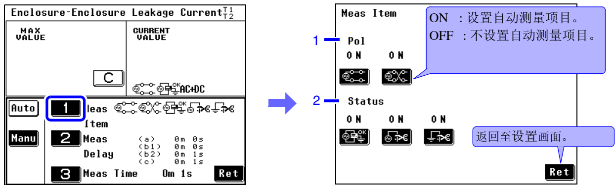
接地泄漏电流测量模式下的自动测量项目
