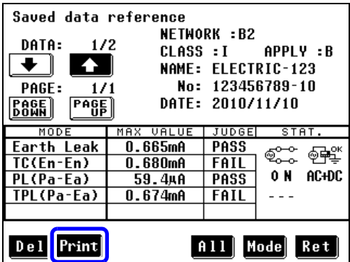
已保存的测量数据参考画面
