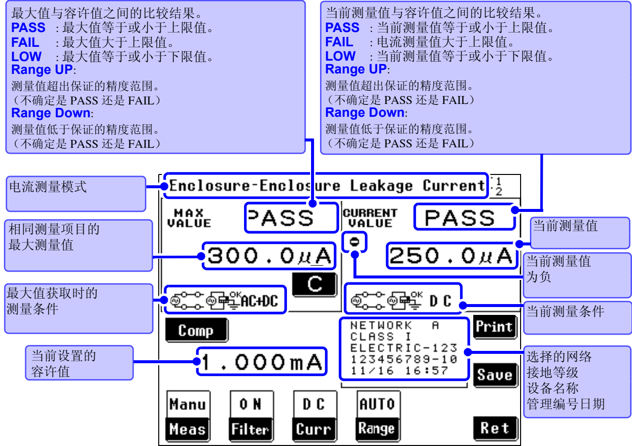
测量画面（手动测量）
