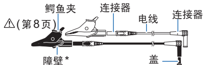
L9257 连接线
