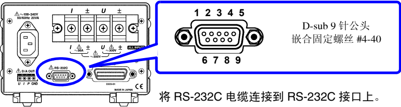
RS-232C 接口
