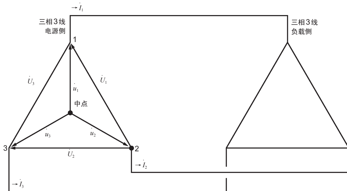
三相3线线路的类似电路
