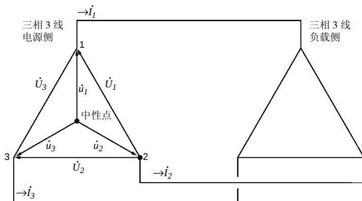
三相 3 线线路的类似回路
