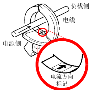
9661 钳式传感器
