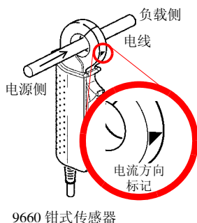
9660 钳式传感器
